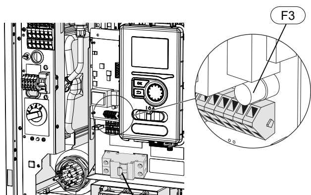
Maalühiskaitse RCD
