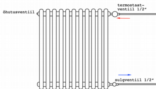
RADIAATORI PÕHIMÖTTELINE ÜHENDUSKEEM ribiradiaator Ercos Comby (küljeltühendus)
