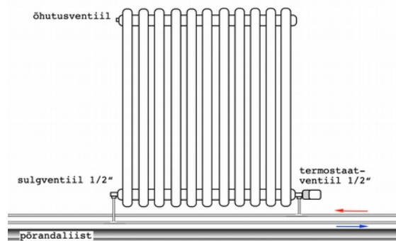
RADIAATORI PÕHIMÖTTELINE ÜHENDUSKEEM ribiradiaator Ercos Comby (torustiku paiknemisel põrandaliistu kohal)
